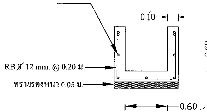
รูปตัด, ขยายเสริมเหล็ก
