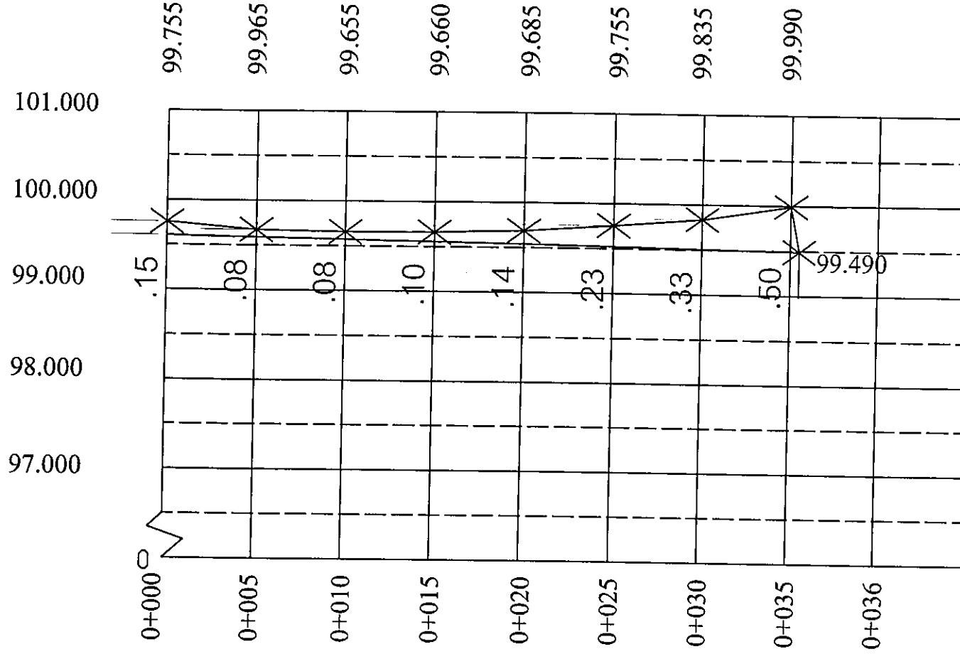
รูปตัดระดับตามยาว
