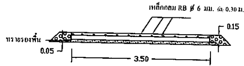
รูปตัดตามขวาง
